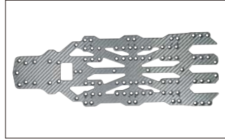
OTA-Zeon カーボンメインシャーシ フロント Mark4 シルバー JAN : 4562226715213 型番 : ZE4001 希望小売価格 : 7,500 円(税別)
